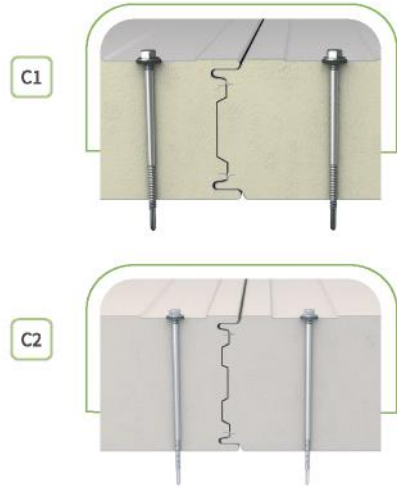
Birleşim Detayı Connection Detail
